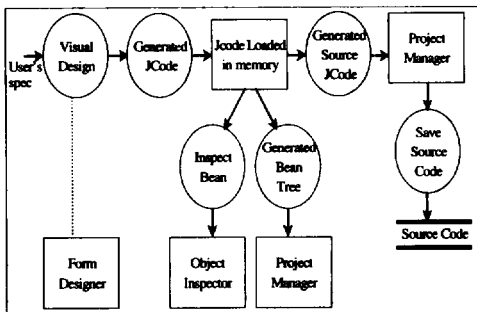
(그림 11) 설계된 IDE에서의 초기화 과정 (Fig. 11) Initialization process in the IDE designed
