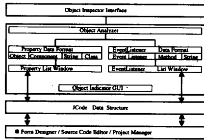
(그림 3) 오브젝트 인스펙터의 구조 (Fig. 3) Architecture of object inspector
