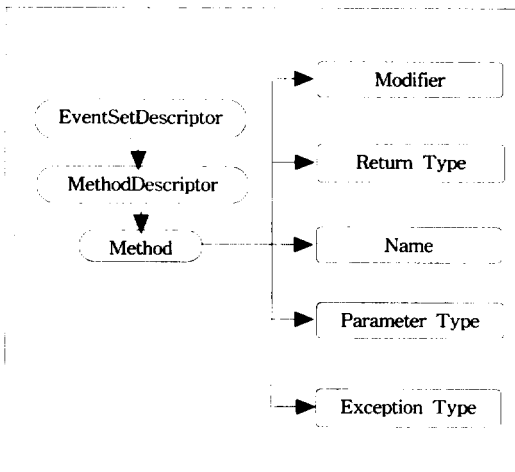
(그림 5) 'EventListener' 메소드의 정보 추출 과정 (Fig. 5) Information extraction process of 'EventListener' method
