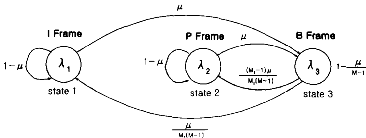
(그림 6) MPEG 비디오 스트림의 3-상태 MMBP 모델 (Fig. 6) 3-State MMBP Model of MPEG Video Stream
