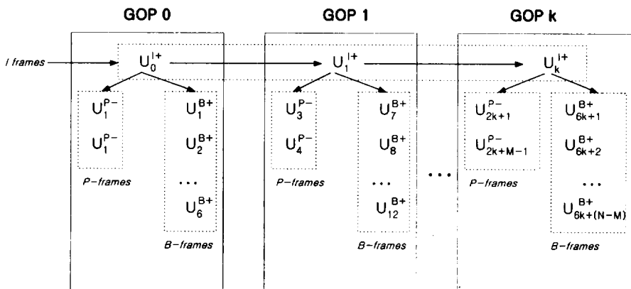
(그림 9) GOP 시퀀스에 관련한 I, P, B 프레임울 위한 background 프로세스의 생성 (Fig. 9) Generation of Background Processes for I, P and B Frames in relation to the GOP Sequence
