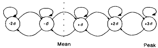
(그림 7) 비디오 소스에 대한 마코브 체인 모델 (Fig. 7) Markov Chain Model for a Video Source
