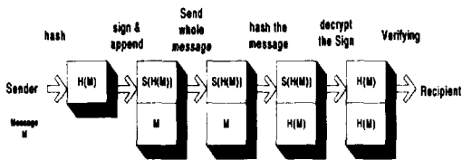
(그림 8) 메시지 서명과 전송 및 인증 구조 (Fig. 8) Stage of digital signature and authentication
