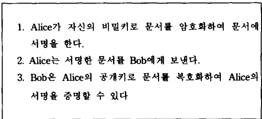
(그림 1) 공개키 방식의 전자 서명 단계 (Fig. 1) Step of digital signature using public key method
