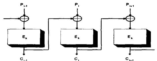
(그림 7) CBC(Cipher block chaining)모드 암호화 방법 (Fig. 7) DES-CBC mode encryption
