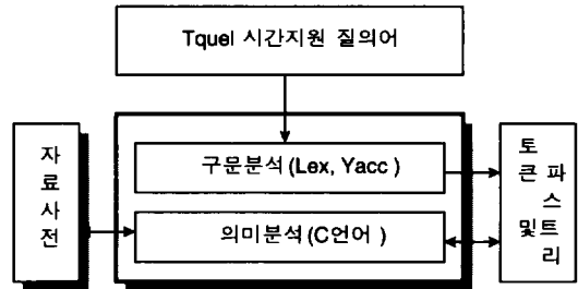
(그림 2) 시간지원 구문분석 및 의미분석 (Fig. 2) Temporal Syntactic and Semantic Analyzer
