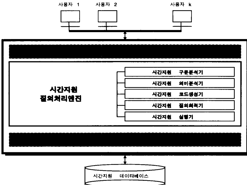
(그림 1) 시간지원 데이터베이스 관리 시스템 구조 (Fig. 1) Architecture of Temporal Database Management System
