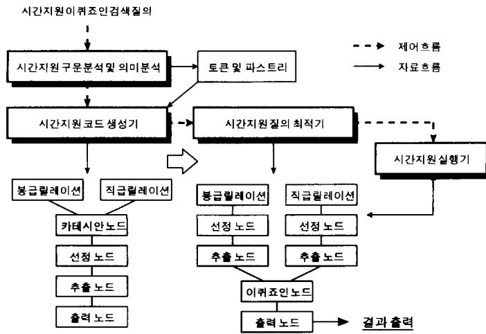
(c) 시간지원 질의처리 과정 (c) Temporal Query Processing
