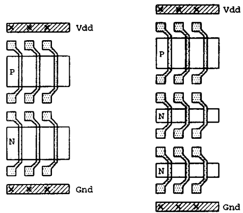
(b) Gate-isolation 구조 [11].
