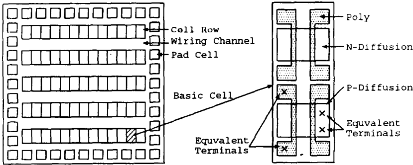
(그림 1) 기초셀을 포함하는 게이트 어레이 구조의 전형적인 예.
