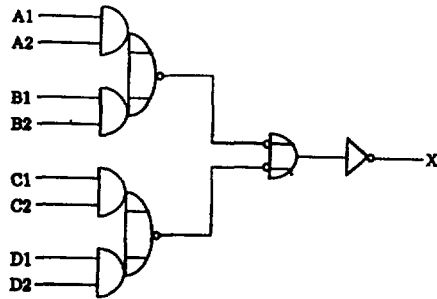
(a) 논리 회로.
