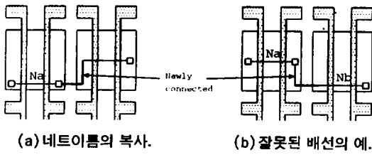
(그림 3) 배선에 따른 넷 이름의 처리.
