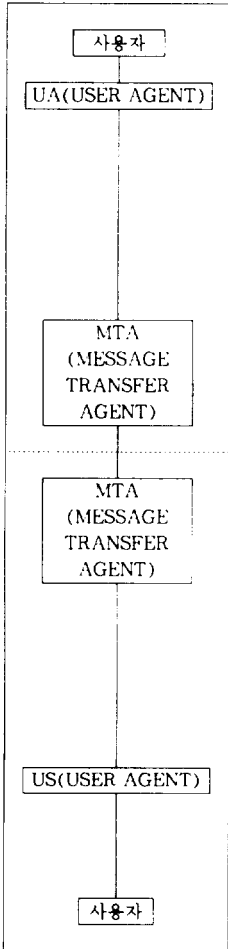
(그림 3) RFC822의 전자우편시스템 (Fig. 3) Mail System in RFC822
