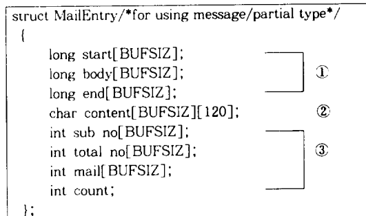
(그림 8) 전자우편 객체를 위한 정보 (Fig. 8) Handling information of "Partial type" Mail
