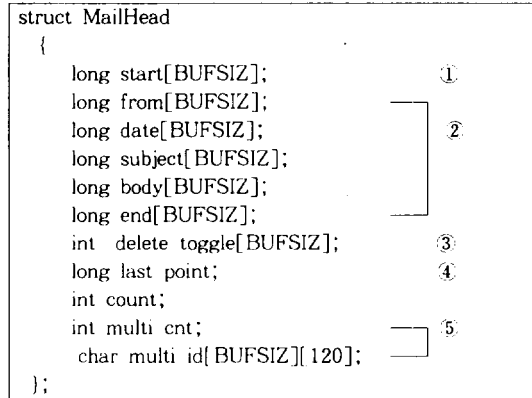
(그림 7) 전자우편 메시지에 대한 정보 (Fig. 7) Handling information of Mail Message
