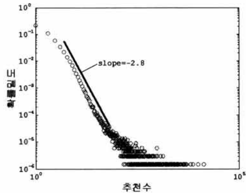
(b) 추천 수 분포
