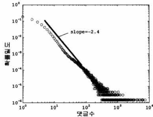
(c) 댓글 수 분포
