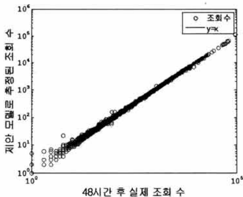
(그림 7) 실제 조회수와 제안 모델로 추정된 값과의 상관관계
