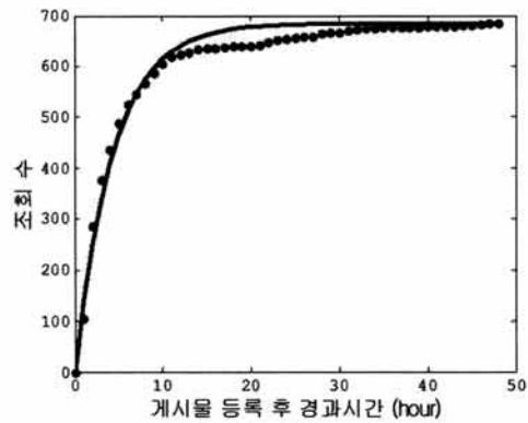
(그림 8) 관찰된 조회수와 제안 모델로 추정된 함수 그래프
