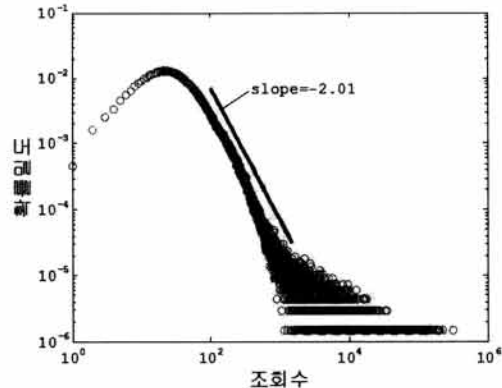
(a) 조회수 분포
