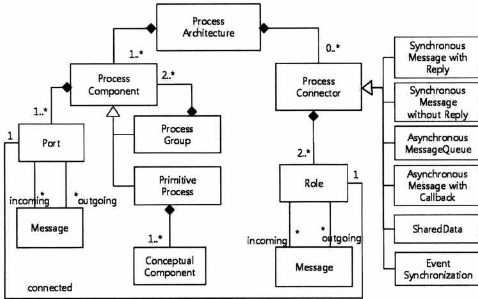
(그림 3) FORM 프로세스 아키텍처 메타 모델
