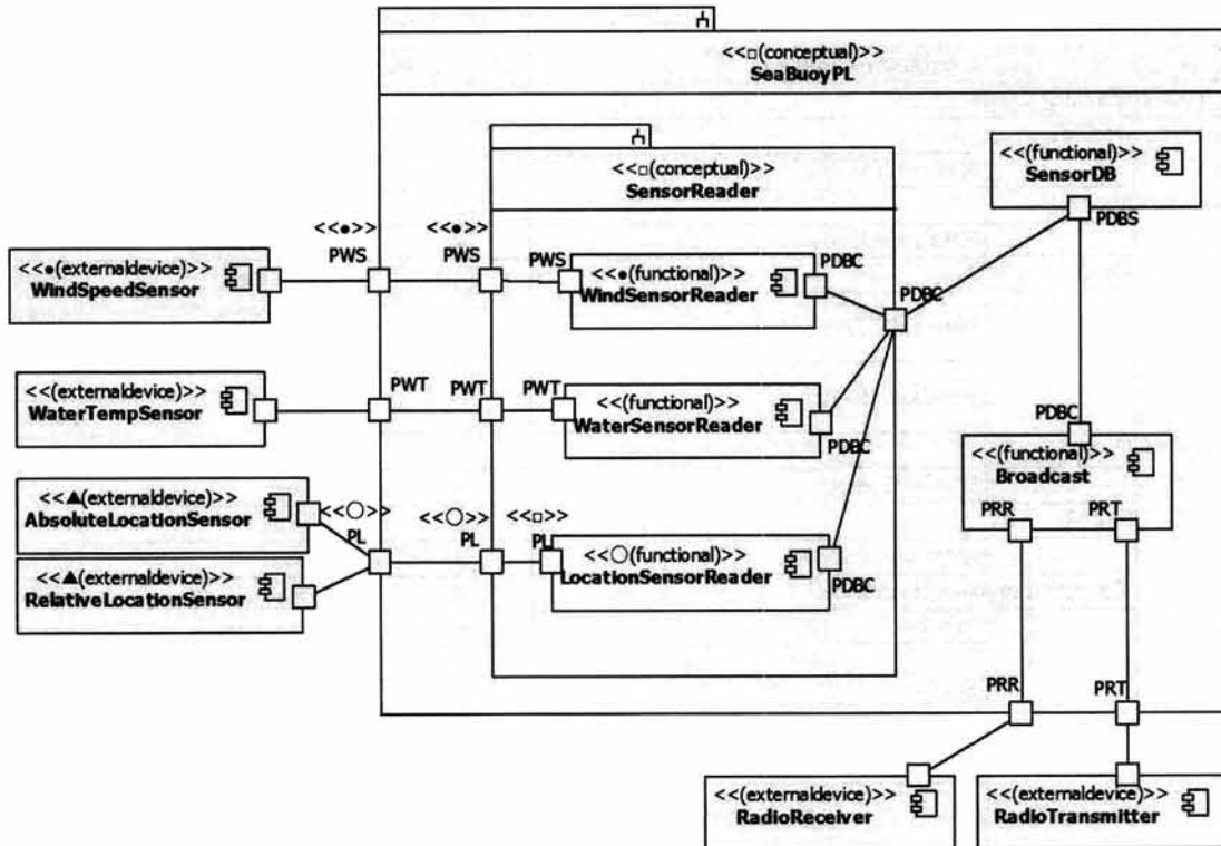
(그림 7) 가변성 적용 후 아키텍처 모델
