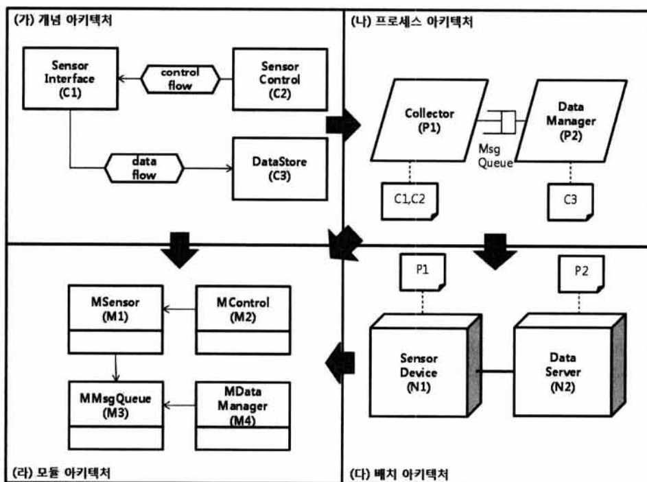
(그림 1) FORM 아키텍처 모델
