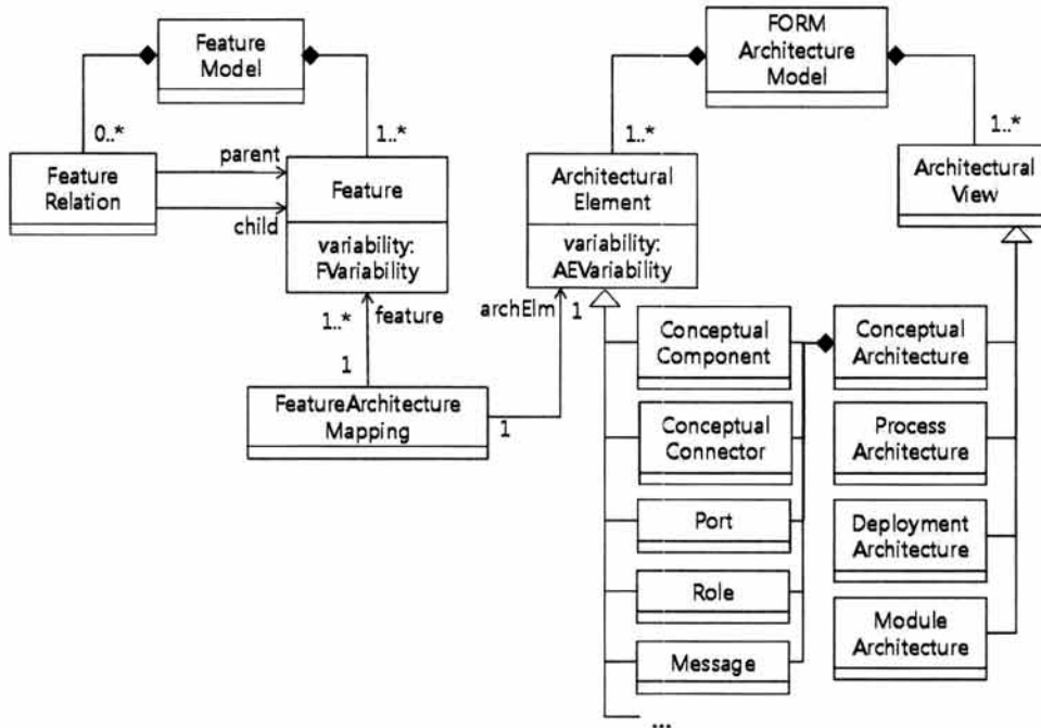
(그림 4) 휘처모델과 FORM 아키텍처 모델의 대응
