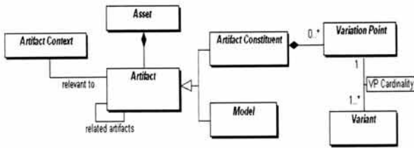
(그림 3) 소프트웨어 프로덕트 라인 자산 메타모델 [7]
