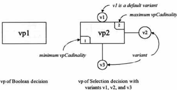
(그림 7) 가변성 의존관계 분석모델 구성요소
