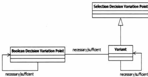
(그림 10) 가변성 의존관계 유형 및 존재관계
