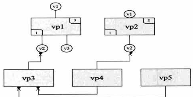
(그림 13) 사례연구(그림 8)에 대한 가변성 의존관계 분석모델
