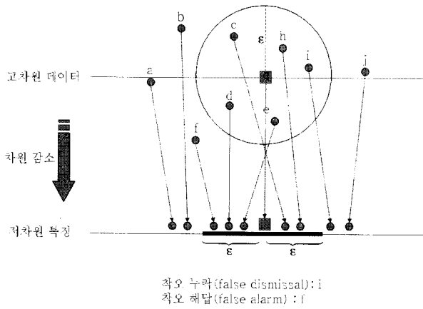
(그림 1) 차원 감소에 의한 착오 누락 및 착오 해당의 예
