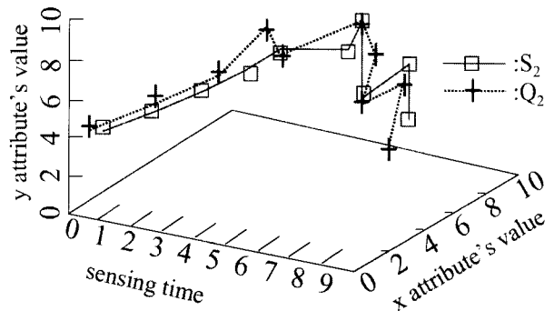
(그림 2) 두 개의 속성을 가진 시퀀스의 예
