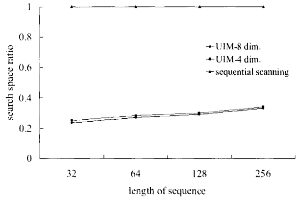
(그림 7) 길이 변화에 따른 3중 속성 시퀀스에서 검색 공간 비율
