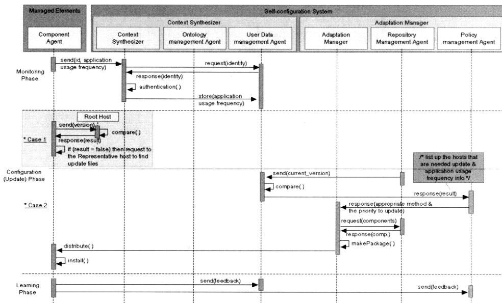
(그림 5) Update 과정의 시퀀스 다이어그램
