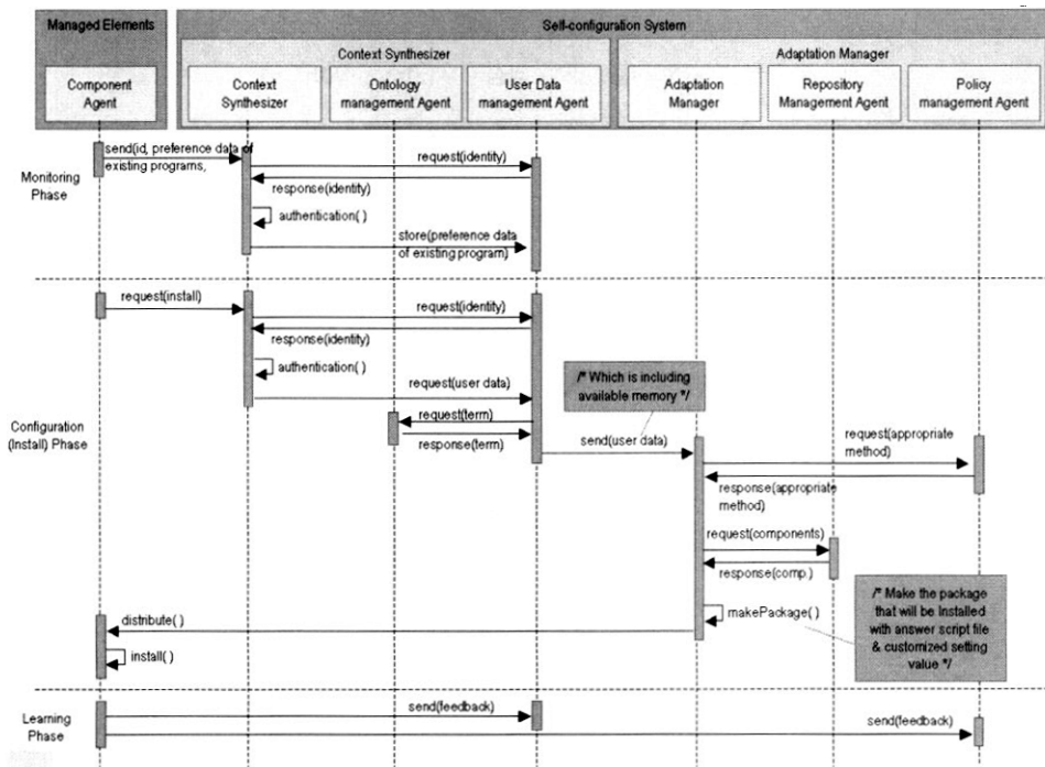
(그림 3) Install 과정의 시퀀스 다이어그램
