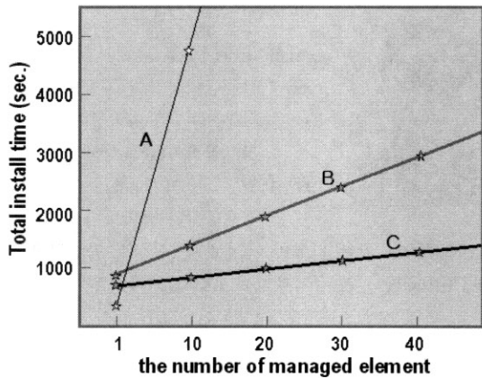
(그림 10) 세 방식의 Install time 비교 그래프
