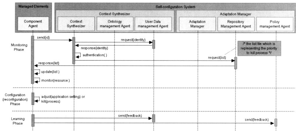
(그림 4) Reconfiguration 과정의 시퀀스 다이어그램
