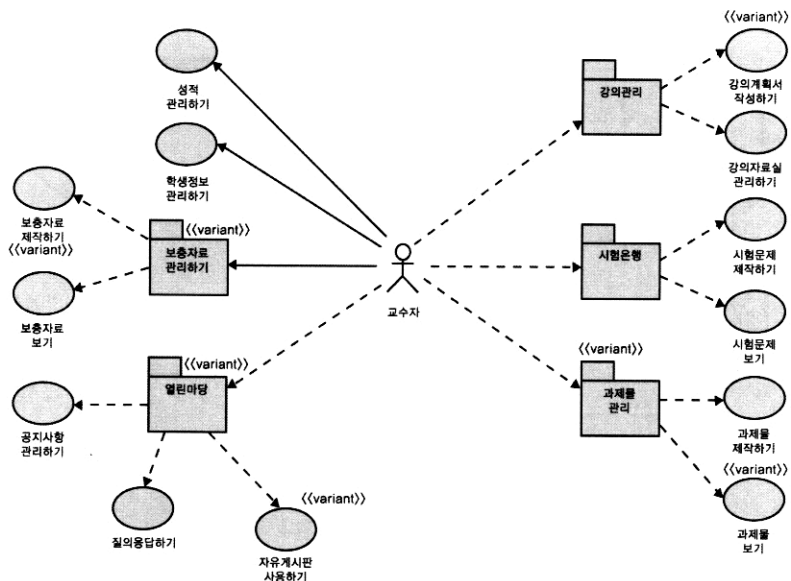
(그림 20) 교수자 시스템의 유스케이스 뷰
