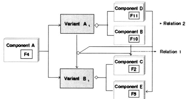
(그림 11) 변화점의 표현
