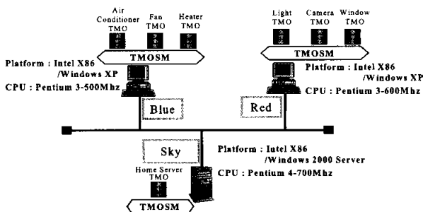
(그림 5) 정보가전 제어 시뮬레이터의 물리적 분산시스템 수행환경
