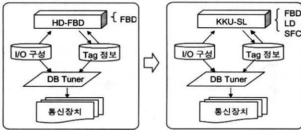
(그림 20) 기존 시스템과의 결합
