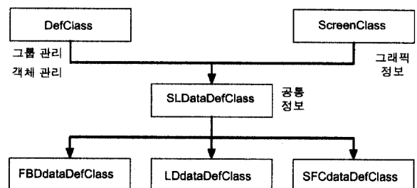
(그림 13) 데이터 구조 처리
