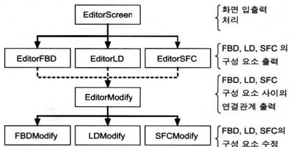
(그림 14) 그래픽 처리
