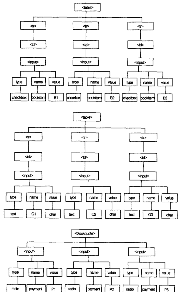
(그림 7) HTML 문서의 계층적 표현
