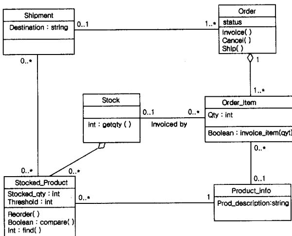
(그림 1) 주문처리 시스템의 클래스 다이어그램
