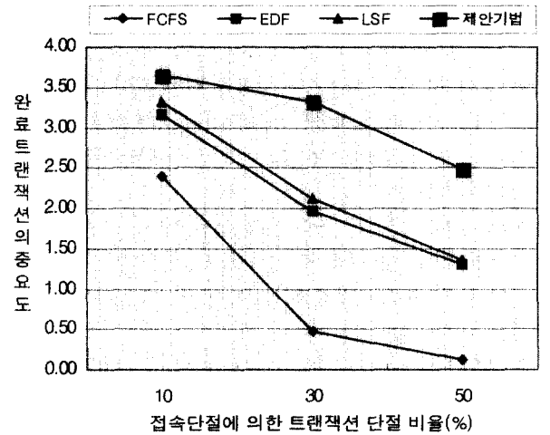
(그림 8) 접속단절에 따른 완료 트랜잭션의 중요도
