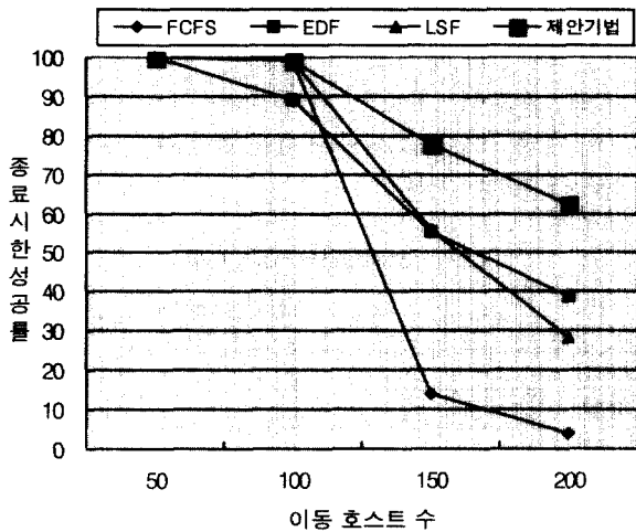
(그림 5) 이동 호스트 수에 따른 스케줄링 기법의 종료시한 성공률
