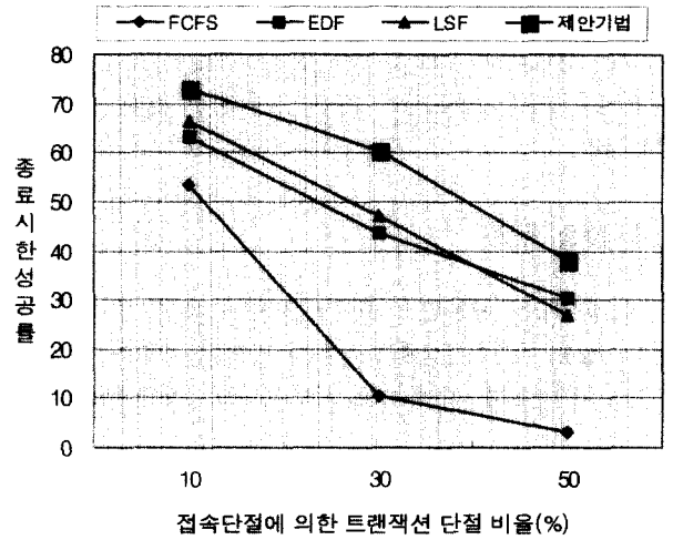
(그림 7) 접속단절에 따른 스케줄링 기법의 종료시한 성공률
