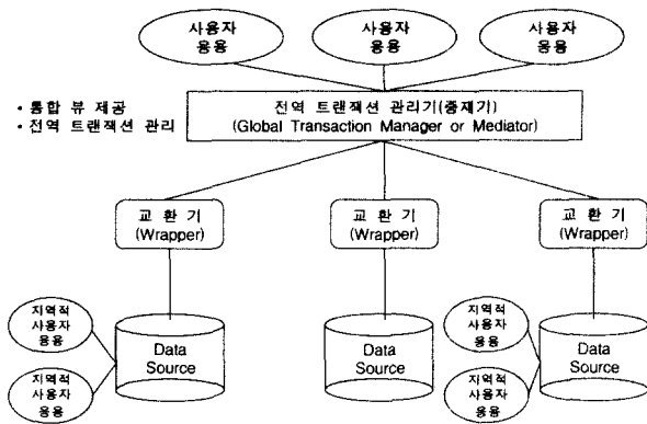
(그림 1) 데이터 통합 시스템 공통 구조
