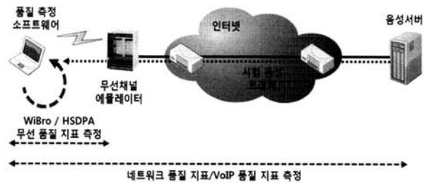
(그림 6) 무선 채널 에뮬레이터를 이용한 실험 환경
