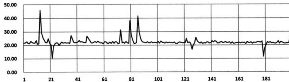
(그림 9) 와이브로를 통한 지터 측정 결과 (설정 3, G.711)
