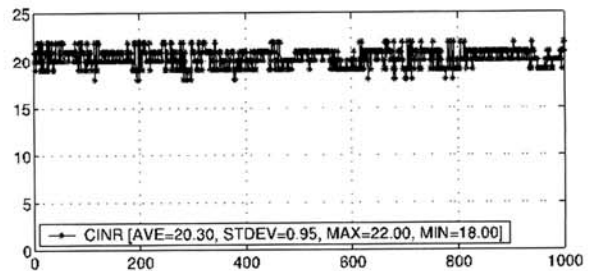
(b) CINR
