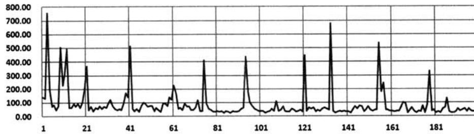
(그림 8) 와이브로를 통한 지연 측정 결과 (설정 3, G.711)
