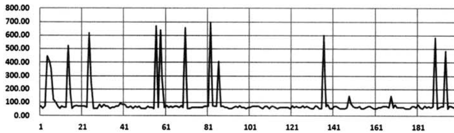
(그림 12) HSDPA를 통한 지연 측정 결과 (설정 3, G.711)
