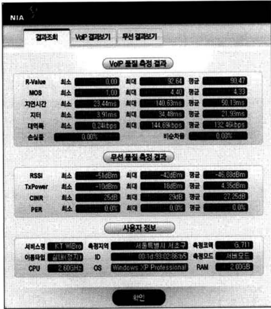
(그림 3) 300초 동안의 측정으로 얻어진 각 품질 지표의 샘플 데이터 예
