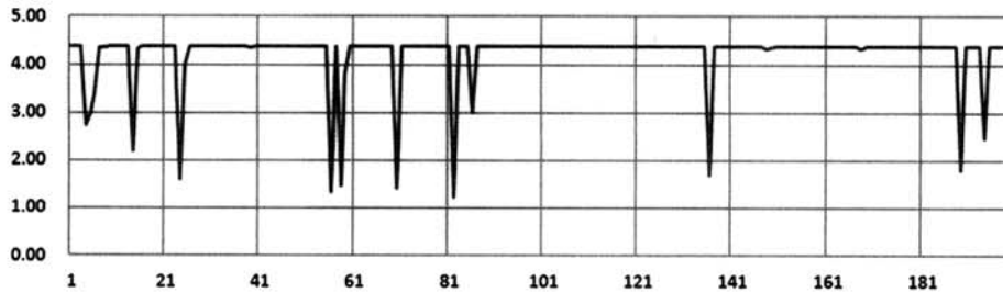
(그림 11) HSDPA를 통한 MOS 측정 결과 (설정 3, G.711)
