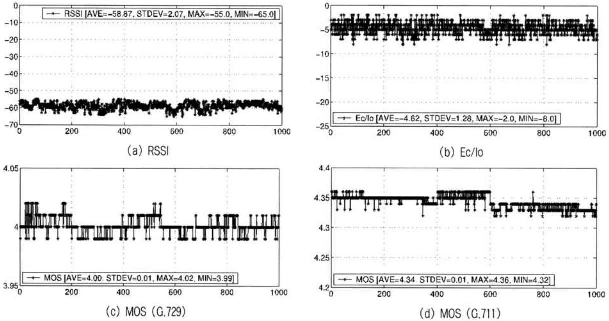
(그림 5) HSDPA를 통한 인터넷 이동 전화 서비스의 품질 측정 결과
