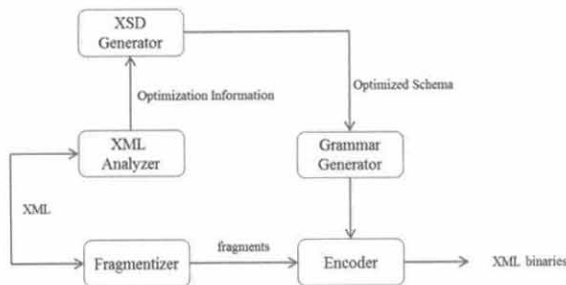
(그림 6) 최적화 정보 기반 EXI 인코딩 구조
