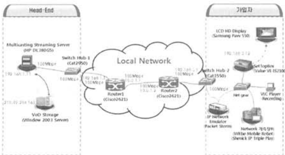
(그림 3) 시험 네트워크 구성 및 장비 설정
