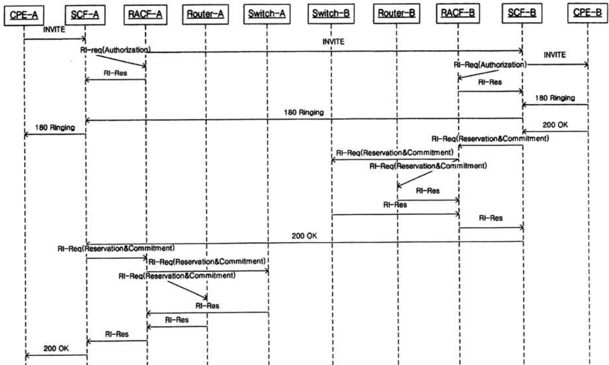
(그림 6) Rs와 Rw 인터페이스의 병행성을 이용한 고속의 두 단계 자원제어 스킴
