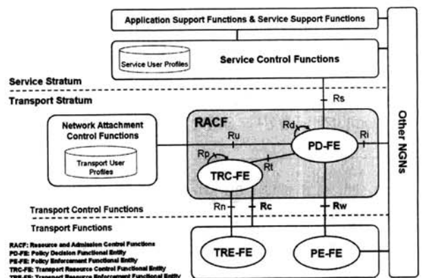
(그림 2) NGN의 기능 구조 및 인터페이스
