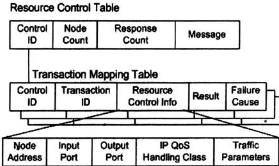
(그림 5) Rw 인터페이스의 자원제어를 위한 자료 구조
