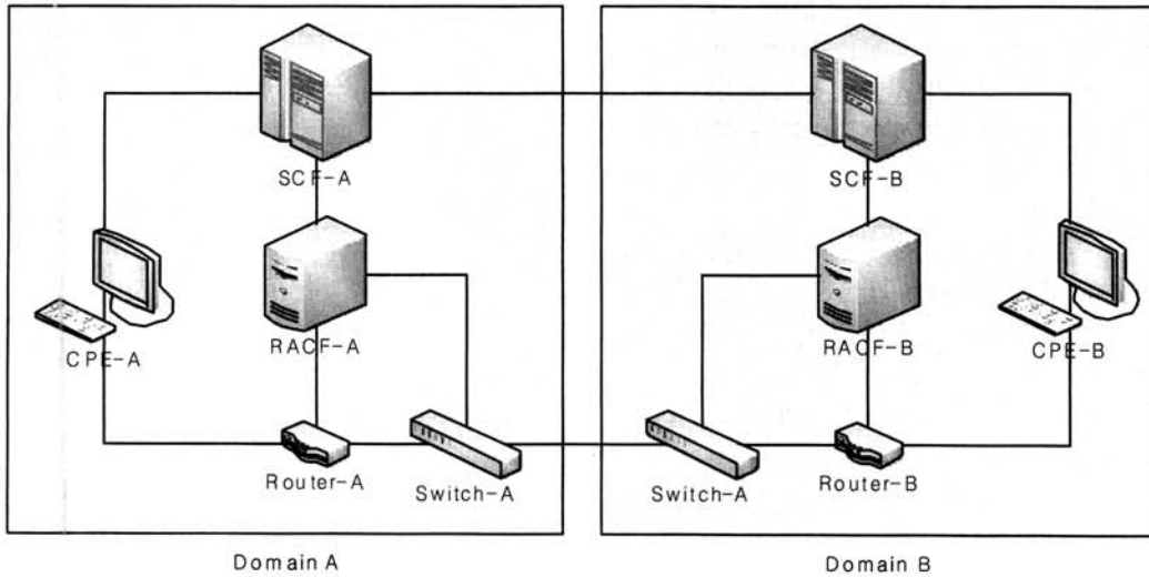
(그림 7) NGN 자원제어 스킴의 시뮬레이션 구성도
