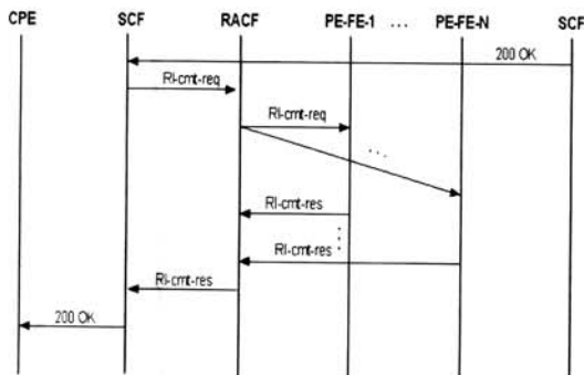
(그림 4) R_w 인터페이스의 병행형 자원제어 절차
