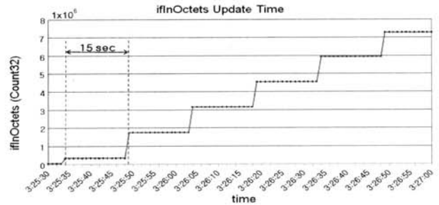
(그림 1) ifInOctets의 갱신 주기
