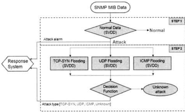
(그림 3) SVDD 기반 탐지 모듈의 계층적 탐지 절차
