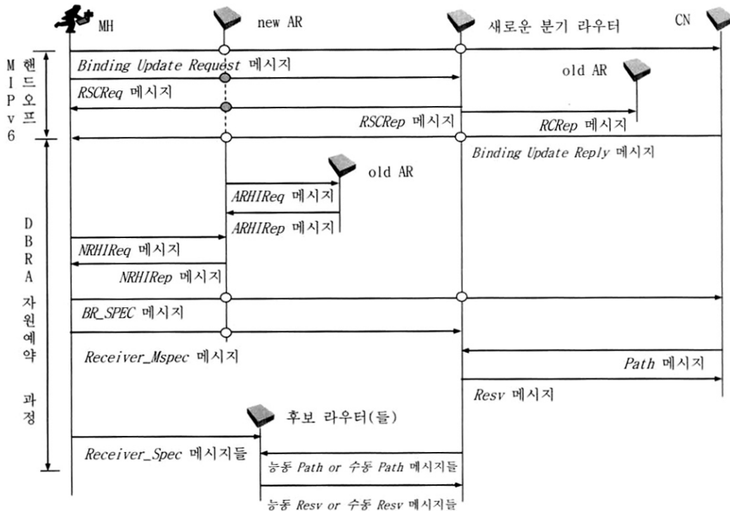
(그림 6) DBRA 메시지 다이어그램
