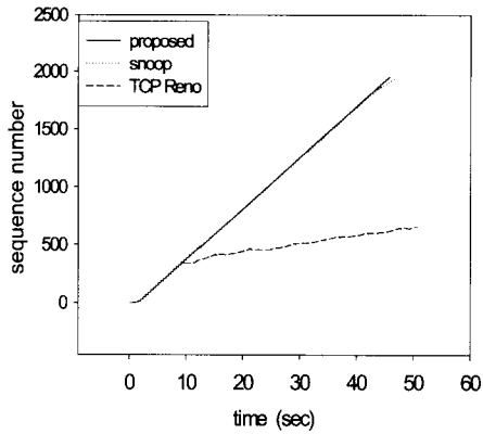
(그림 7) 이동 호스트에 도착한 시퀀스 번호 (MBP = 4 msec, 두 개의 무선링크)
