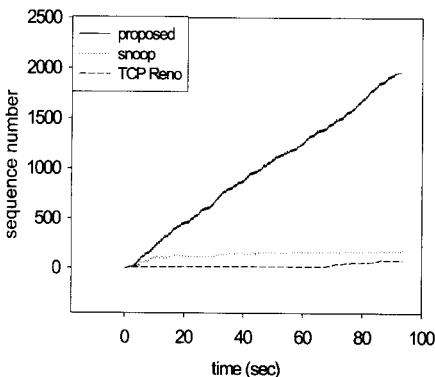
(그림 9) 이동 호스트에 도착한 시퀀스 번호 (MBP = 128 msec, 두 개의 무선링크)
