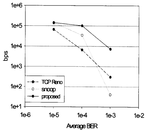
(그림 12) BER에 따른 throughput 비교 (네개의 무선링크)
