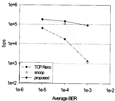
(그림 10) BER에 따른 throughput 비교 (두개의 무선 링크)
