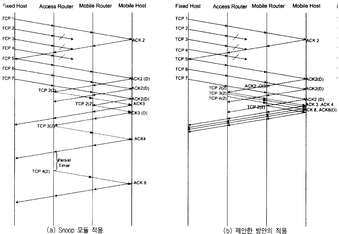
(그림 5) Snoop과 제안 모듈에서 연속된 패킷 손실에 대한 처리 비교
