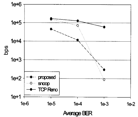
(그림 11) BER에 따른 throughput 비교 (세개의 무선링크)
