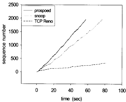
(그림 8) 이동 호스트에 도착한 시퀀스 번호 (MBP = 32 msec, 두 개의 무선링크)
