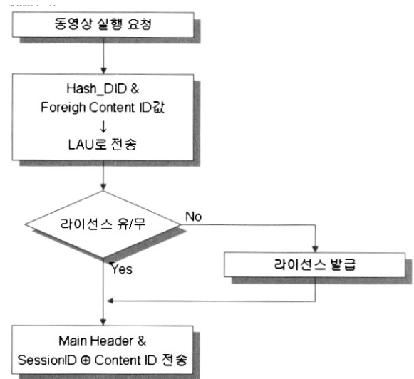
(그림 10) 복호화 전처리 작업
