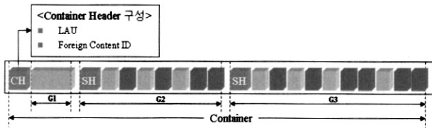
(그림 8) 전체 동영상의 Container와 Container 헤더
