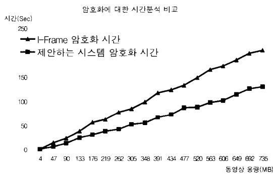
(그림 15) 암호화에 대한 시간분석 비교 그래프
