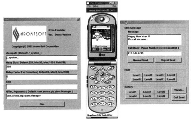
(그림 1) 아로마 위피 에뮬레이터
