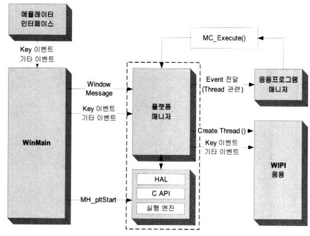
(그림 5) CNU 위피 에뮬레이터 내부 기능 구조
