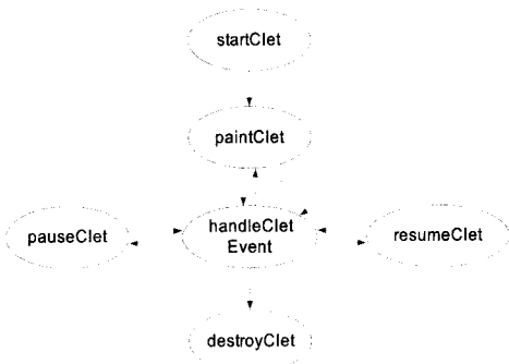
(그림 6) 위피 응용프로그램 생명 주기
