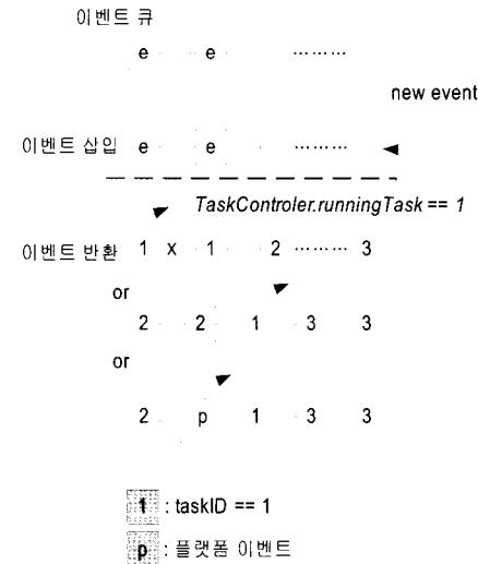
(그림 11) 실행엔진 2.0의 이벤트 큐 동작
