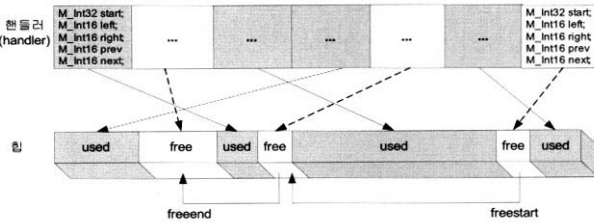
(그림 10) 메모리 관리자를 위한 자료구조 사용
