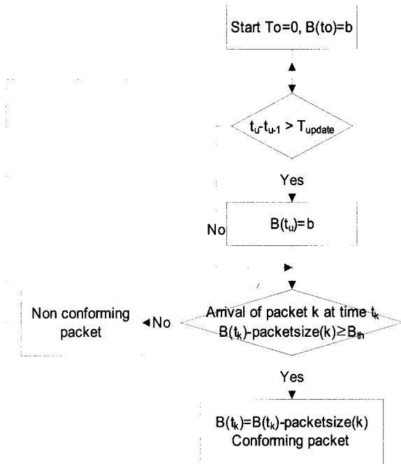
(그림 5) 레이트 제한 알고리즘
