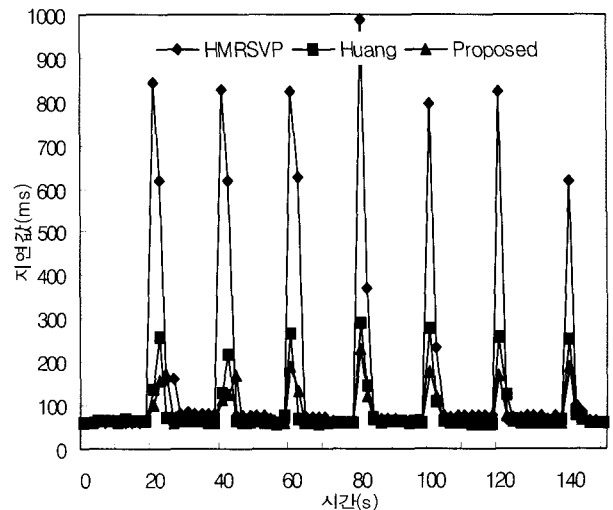
(그림 14) 패킷전달지연
