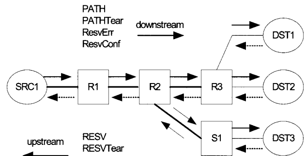
(그림 2) RSVP 메시지
