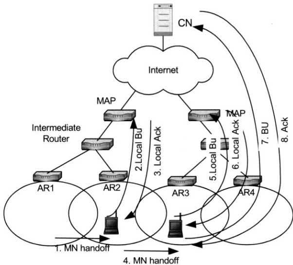
(그림 1) HMIPv6에서 MN의 이동 및 등록
