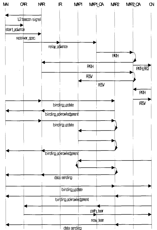
(그림 10) 지역간 이동에서의 메시지 플로우
