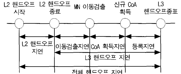
(그림 6) Mobile IPv6의 핸드오프 지연
