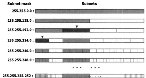
(그림 6) 서브넷 할당 2단계
