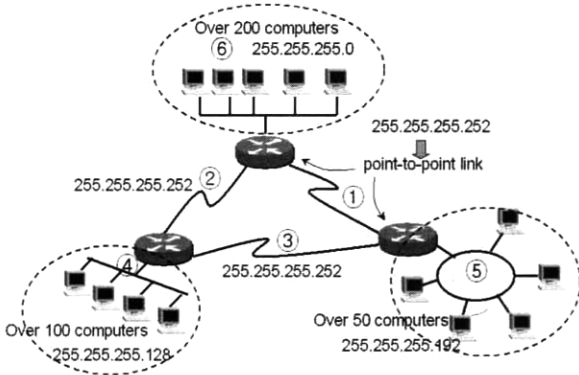
(그림 2) 다양한 규모의 서브넷 예
