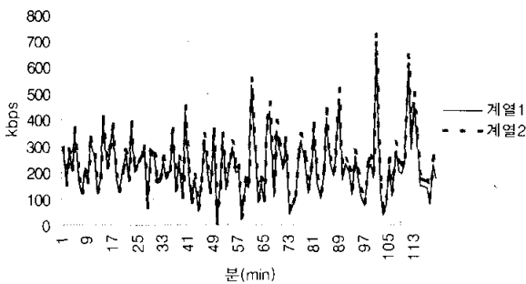
(그림 2) 핸드오프호의 자원요구량(계열1)과 기존의 방법에 의한 자원의 예측량(계열2, \alpha=0.018 )
