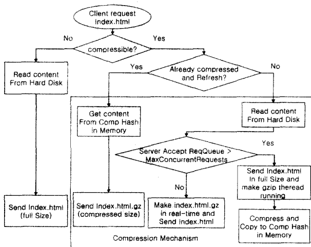
(그림 2) 실시간 압축전송 알고리즘도
