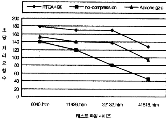
(그림 3) 테스트 파일 사이즈별 서버측의 초당 처리 요청수
