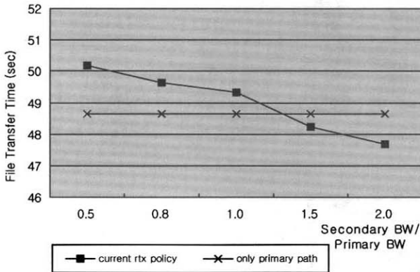
(그림 5) 프라이머리 경로는 4%의 패킷 손실율, 대체 경로는 2%의 패킷 손실율을 가지는 경우, 대체 경로의 대역폭 변화에 따른 지연
