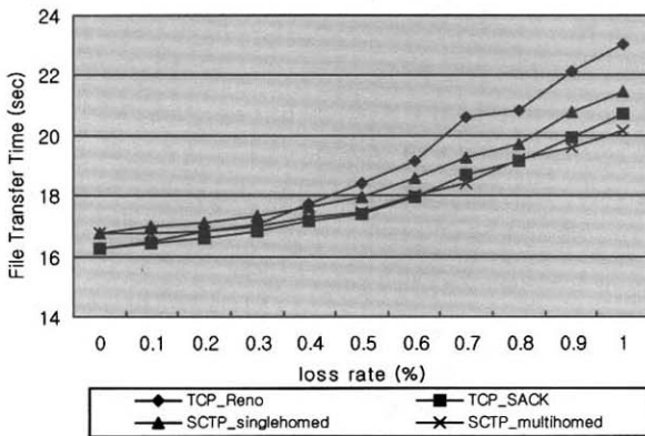
(그림 2) 4MB file 전송시 패킷 손실율에 따른 지연
