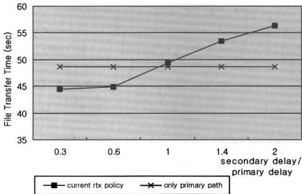
(그림 6) 프라이머리 경로는 4%의 패킷 손실율, 대체 경로는 2%의 패킷 손실율을 가지는 경우, 대체 경로의 전파 지연 변화에 따른 지연
