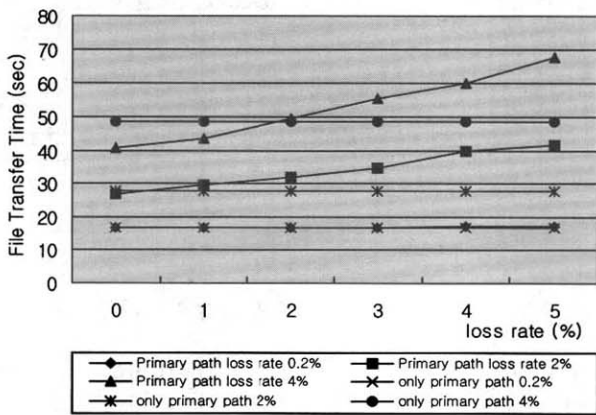
(그림 4) 대체 경로의 패킷 손실율에 따른 지연
