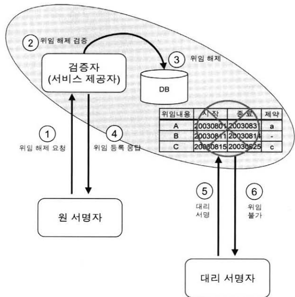
(그림 4) 위임해제 프로토콜 시나리오
