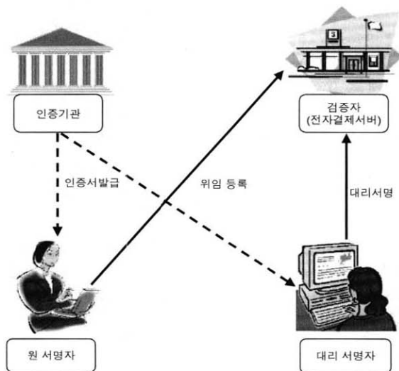
(그림 1) 대리서명 방식의 구성요소
