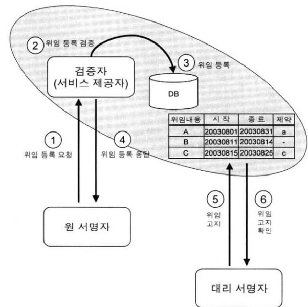
(그림 2) 위임등록 프로토콜 시나리오
