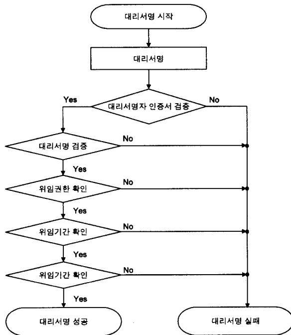
(그림 6) 대리서명 알고리즘
