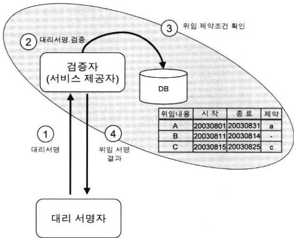
(그림 3) 대리서명 및 검증 시나리오
