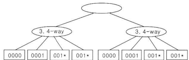
(그림 3) 단계 압축 트라이
