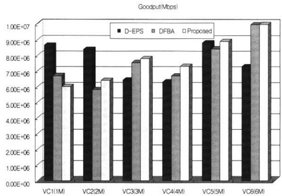
(그림 4) TCP Goodput 비교(VC의 MCR이 다를 경우, MCR의 합 = 21Mbps)
