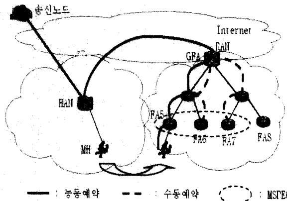
(그림 4) MH가 외부 네트워크에 위치해 있을 때의 자원예약 경로
