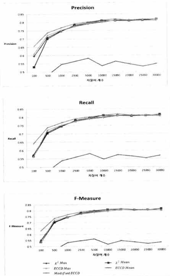
그림 3. Modified ECCD 실험 결과 Fig. 3. Experimental results of Modified ECCD
