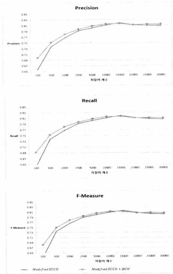
그림 4. 문서별 범주 가중치 검증 실험 Fig. 4. Experiments of category weight for each document
