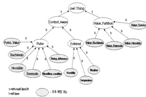
(그림 8) 온톨로지의 클래스 계층 구조
