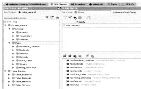
(그림 9) 맥 정보의 온톨로지를 구축한 모습
