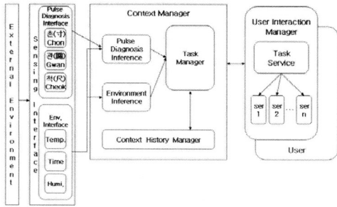
(그림 5) OMPD-CAM의 구조
