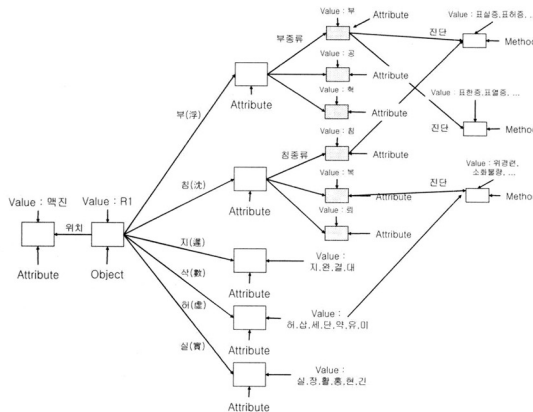
(그림 6) OMPD-CAM의 가상 공간 모델
