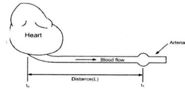
(그림 3) 맥과 전달 속도의 측정
