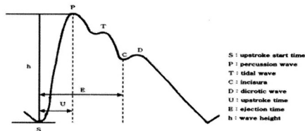
(그림 2) 정상적인 맥파형
