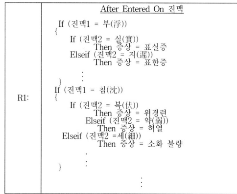
(그림 7) 맥의 규칙 알고리즘
