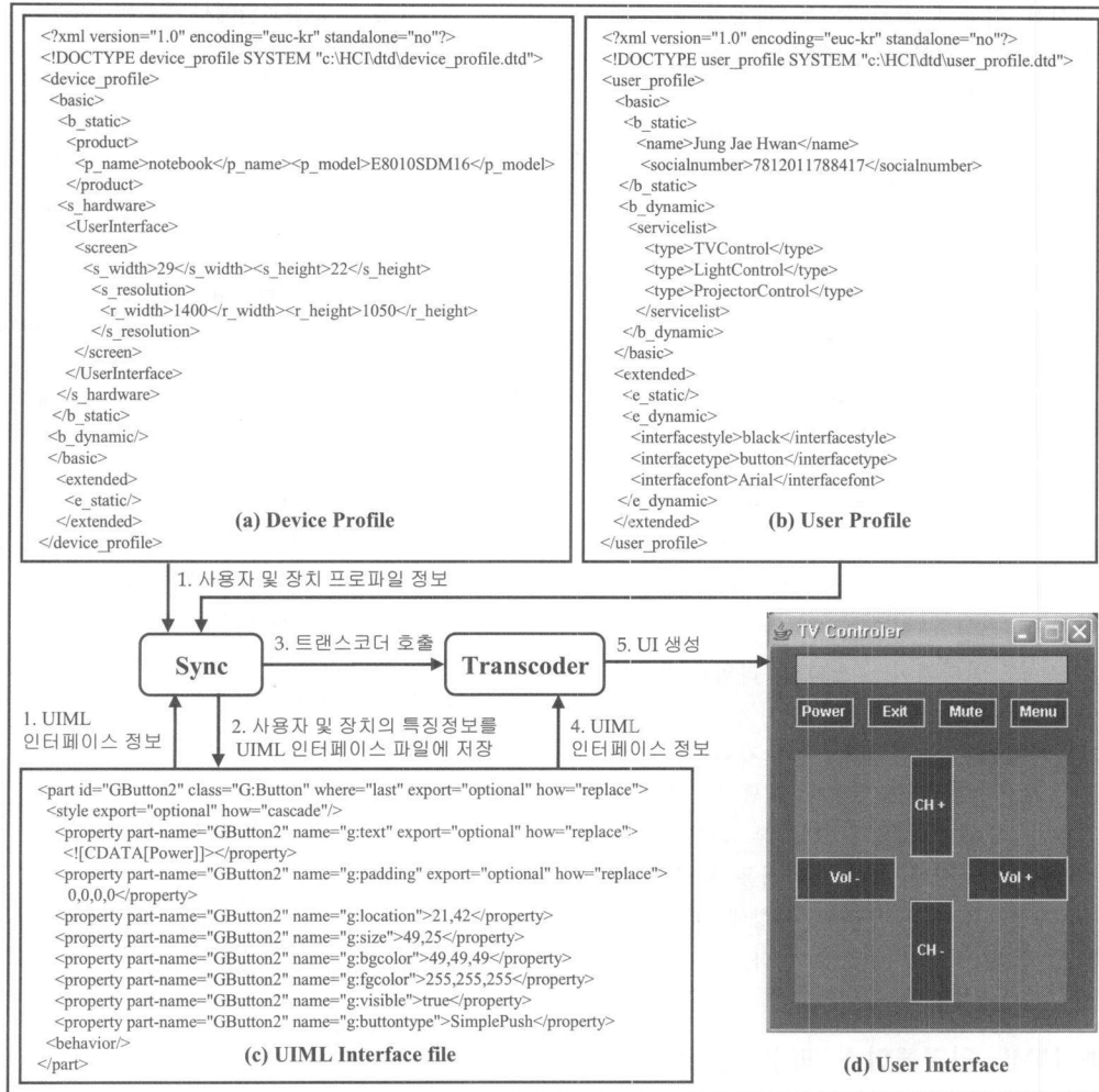
(그림 4) 사용자 인터페이스 생성 과정
