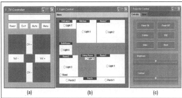
(그림 5) JAVA 기반의 적응형 사용자 인터페이스
