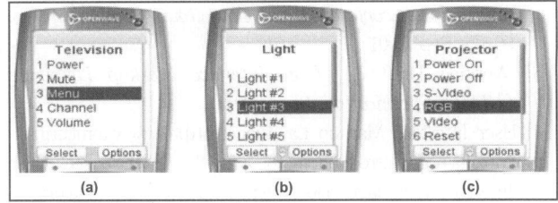
(그림 6) WML 기반의 적응형 사용자 인터페이스
