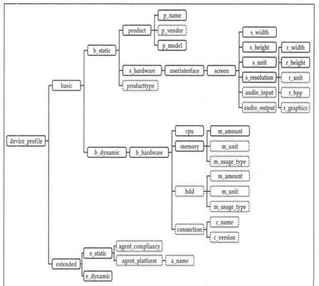
(그림 3) 장치 프로파일 구조
