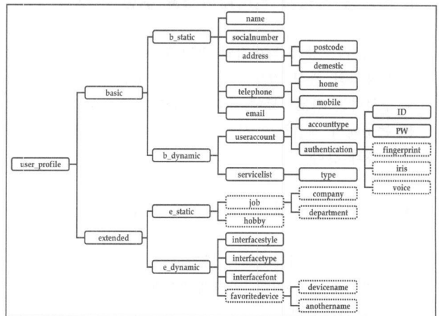
(그림 2) 사용자 프로파일 구조
