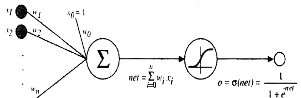
(그림 3) 시그모이드 단위(Sigmoid Unit)의 구조
