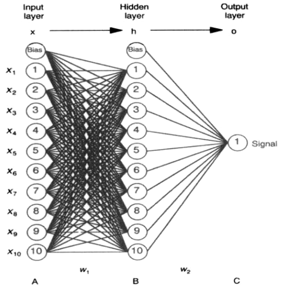
(그림 2) 인공 신경망의 전체 구조
