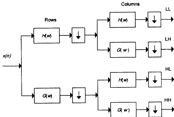
(a) 분해 필터
