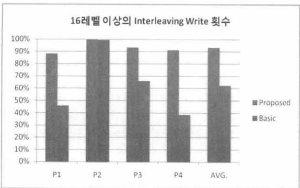
(그림 7) 기존 구조와 제안하는 구조의 Interleaving 효율 비교
