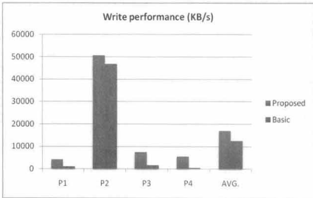
(그림 5) 기존 구조와 제안하는 구조의 쓰기 성능 비교
