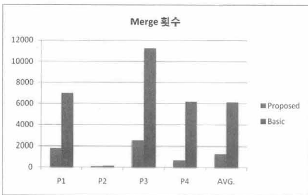
(그림 6) 기존 구조와 제안하는 구조의 병합(Merge) 동작 발생 횟수
