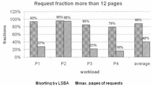
(그림 1) LSBA별로 누적 작성 페이지양과 쓰기 요청당 페이지수의 비교
