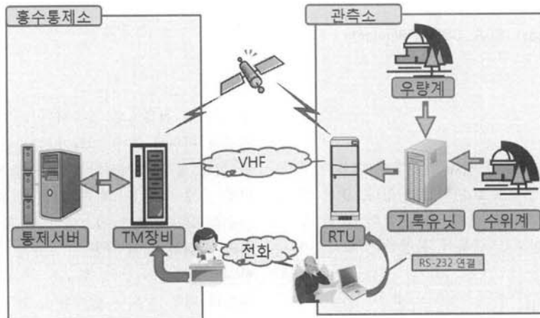
(그림 1) 홍수예보시스템 구성도
