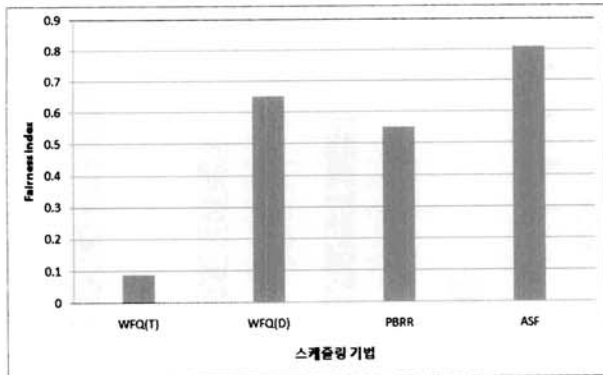
(그림 12) 스케줄링 기법별 Fairness Index
