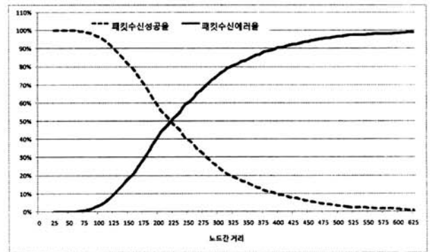
(그림 3) 노드간 거리에 따른 통신 에러율 및 패킷 수신율
