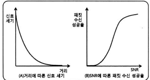
(그림 2) 거리에 따른 신호세기와 SNR에 따른 패킷 수신 성공률
