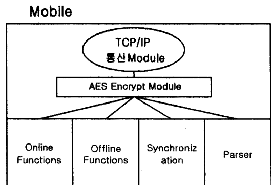
(그림 5) 영업 및 관리자의 Mobile 구조
