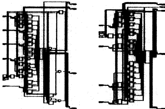
a. Guo 곱셈기 b. 본 연구에서 제안한 곱셈기 (그림 9) (그림 8)에 있는 각각의 PE 회로도
