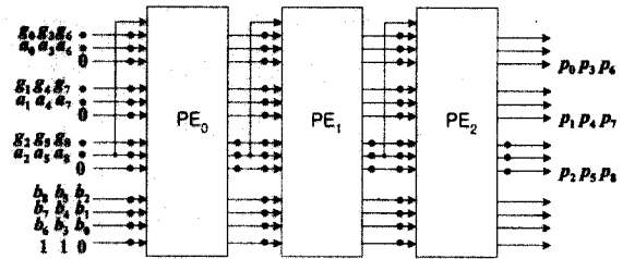
(그림 4) L=3 일 때 GF(2^9) 의 디지털 시리얼 곱셈기 구조
