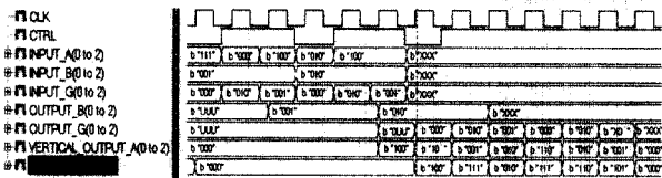
(그림 11) 본 연구에서 제안된 곱셈기에 대한 시뮬레이션 결과
