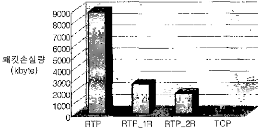
(a) 패킷손실량
