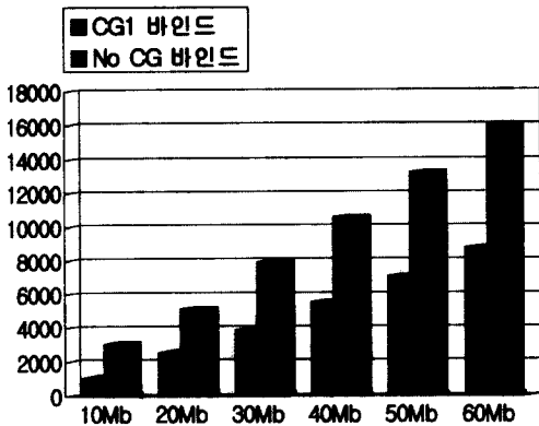
(그림 6) 원격 메모리 접근 횟수 비교
