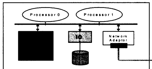
(그림 6) 테스트베드 시스템 구성
