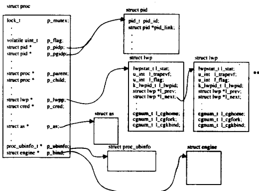
(그림 3) 프로세스 자료구조
